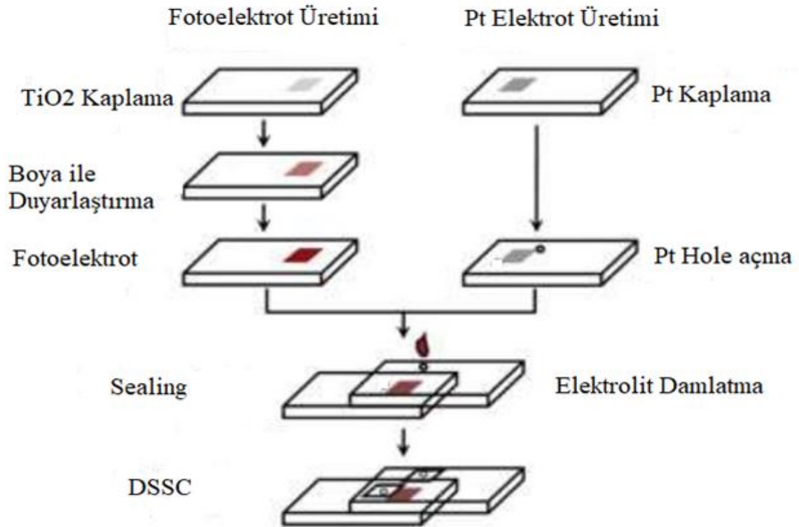
Şekil 3.2. Esnek DSSC Üretim Aşamaları
