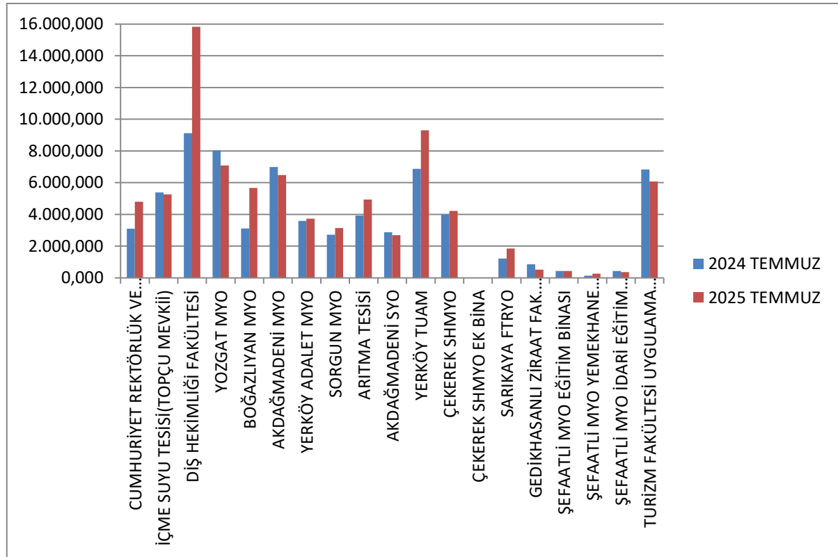
Grafik-4: Abonelik Bazında Elektrik Tüketiminin Temmuz 2024 - Temmuz 2025 Karşılaştırması(Merkez Kampüs Dışı)
