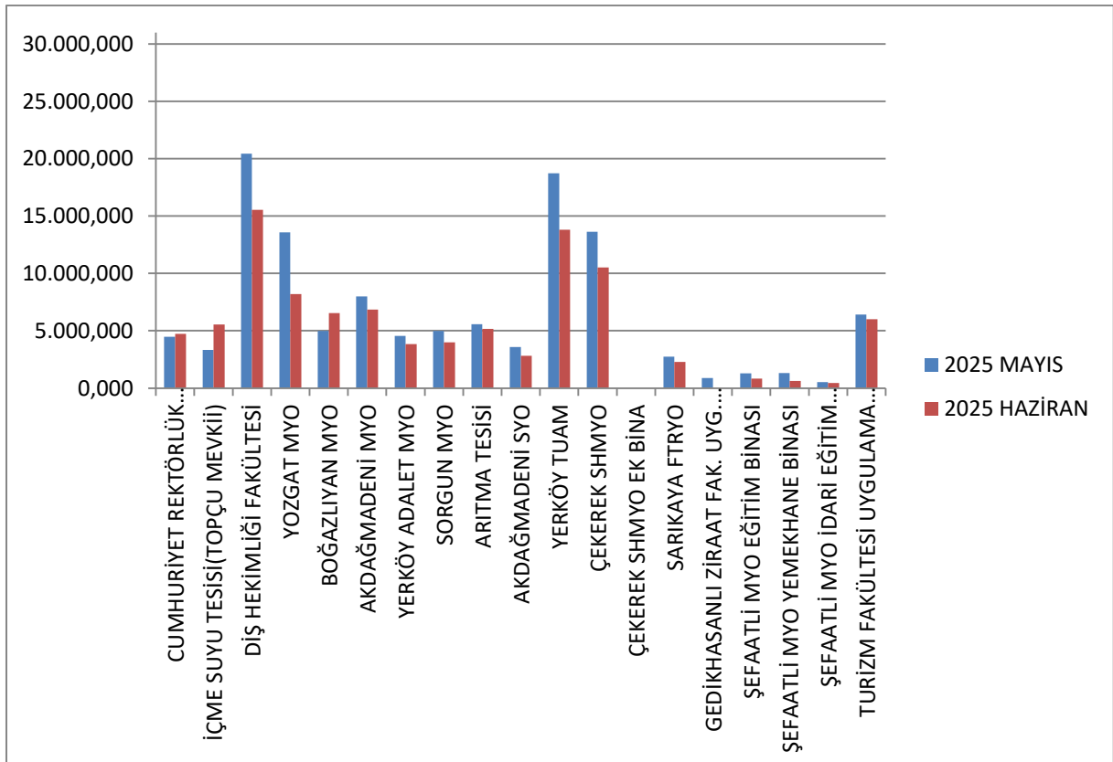
Grafik-2: Abonelik Bazında Elektrik Tüketiminin Mayıs 2025-Haziran 2025 Karşılaştırması(Merkez Kampüs Dışı)
