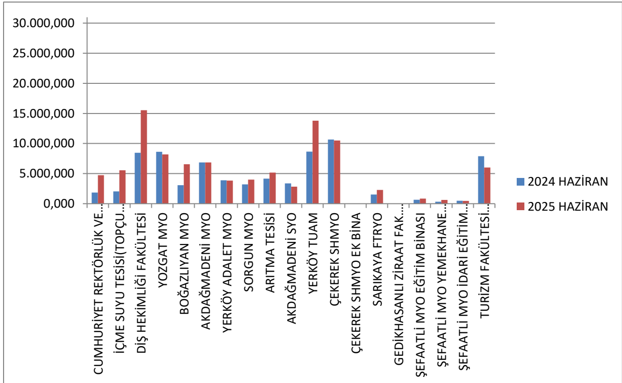
Grafik-4: Abonelik Bazında Elektrik Tüketiminin Haziran 2024 - Haziran 2025 Karşılaştırması(Merkez Kampüs Dışı)
